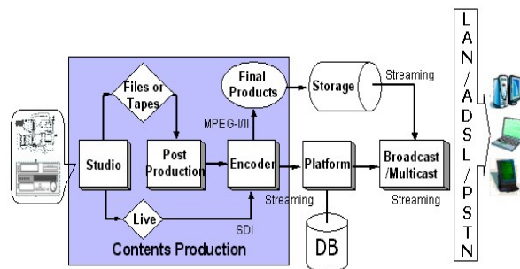
圖 1 架構及流程示意圖
