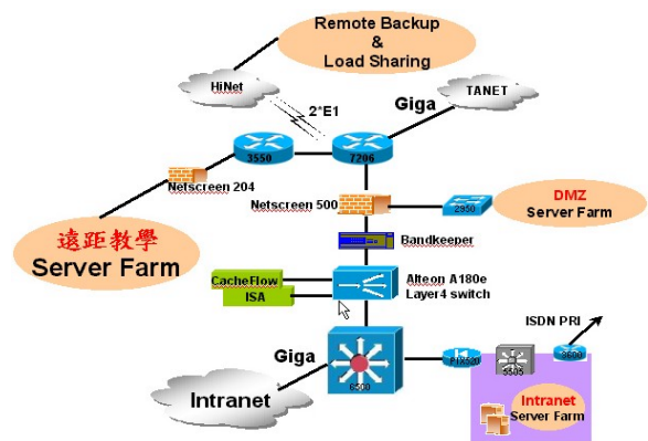
圖 7 網路架構示意圖
