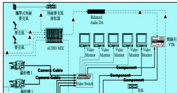
圖 3 攝影棚訊號圖
