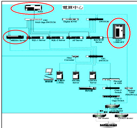
圖 8 伺服器群部署圖
