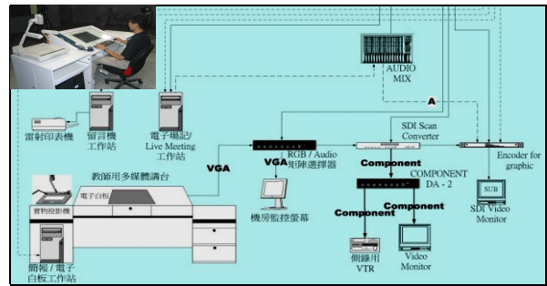
圖 2 多媒體講桌訊號圖
