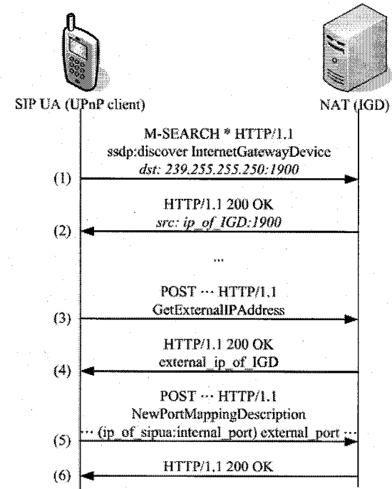
圖 6 UPnP 協調 IP 位址及通訊埠流程
