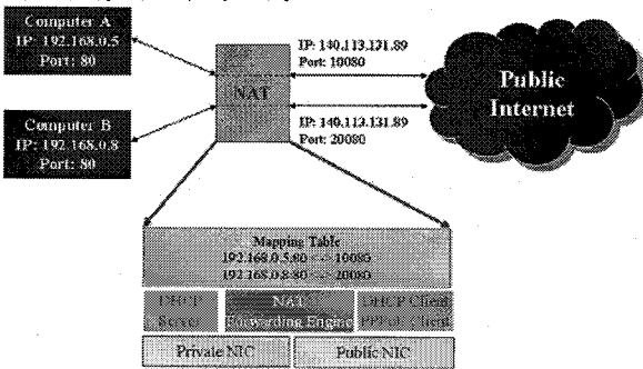
圖 2 NAT 架構圖
