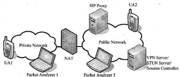
圖 1 測試環境
