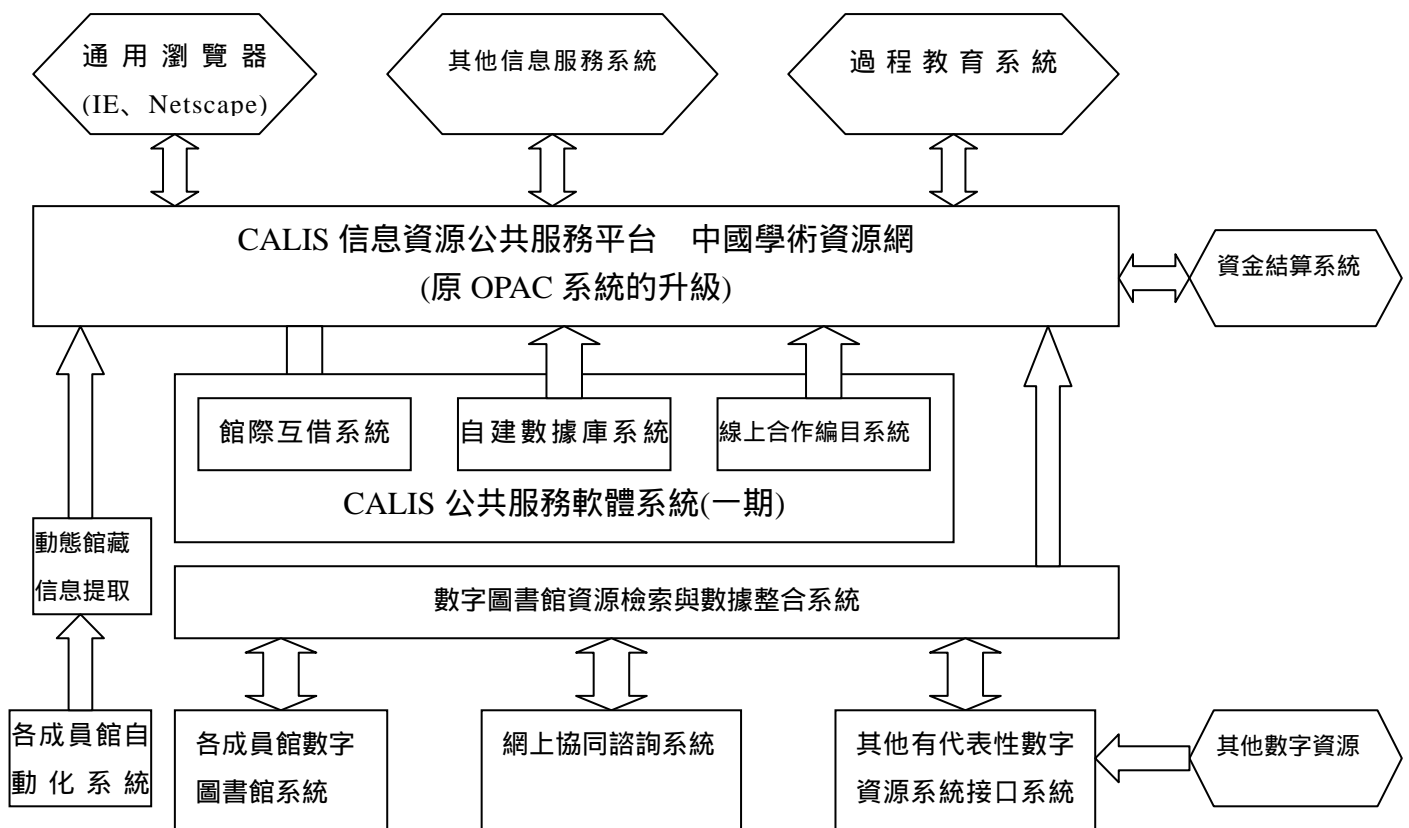
圖 5-5 CALIS 資訊資源公共服務平台架構
