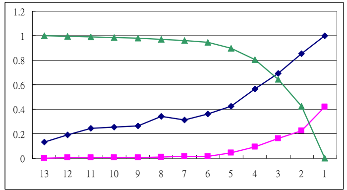
2003 4Q → 4 群
