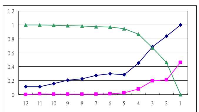
2003 4Q → 4 群
