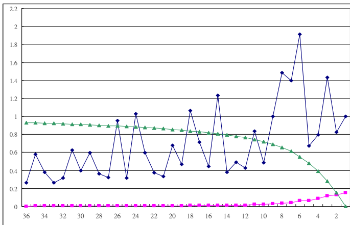
2003 3Q → 6 群
