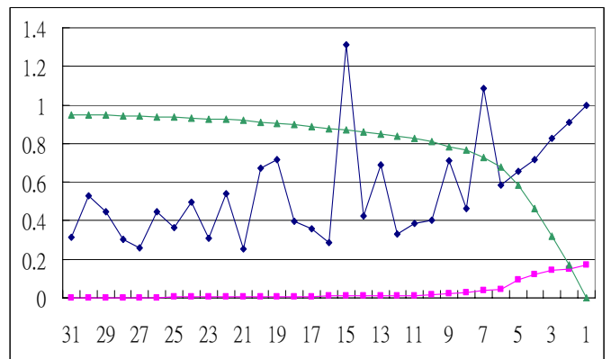
2003 Q → 6 群
