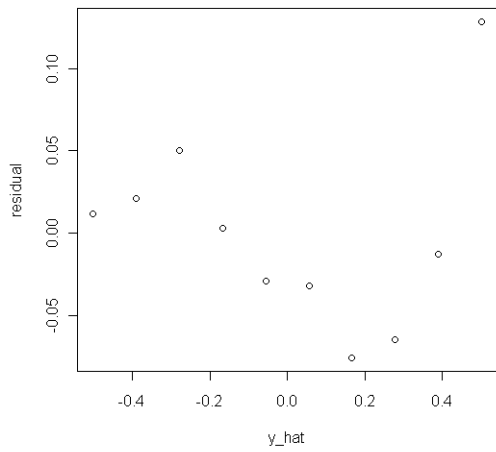
AR(男_年代) : 配適値 vs 殘差
