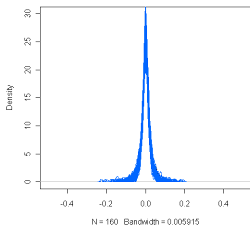
男性ie-100次模擬的殘差機率密度函數
