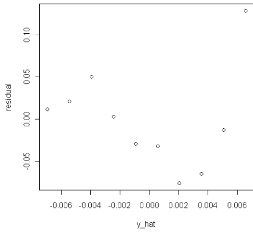
ACP(男_年代) : 配適値 vs 殘差
