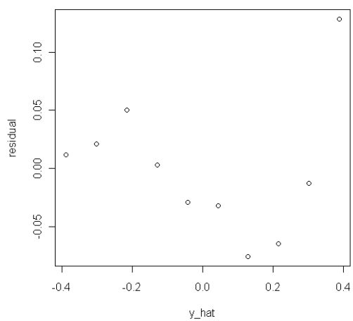
IE(女_年代) : 配適値 vs 殘差
