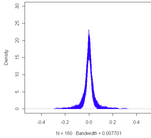
女性cglm_c-100次模擬的殘差機率密度函數
