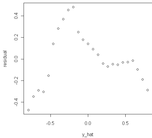
IE(男_世代) : 配適値 vs 殘差
