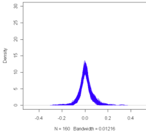
女性acp-100次模擬的殘差機率密度函數
