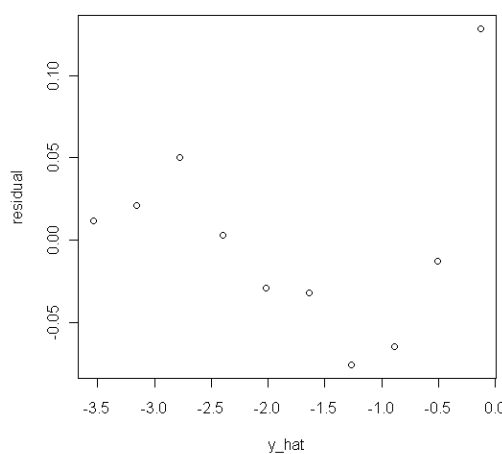
cglim_p(女_年代) : 配適値 vs 殘差
