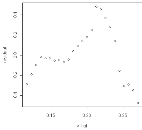
AR(男_世代) : 配適値 vs 殘差
