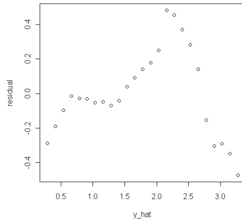
cglm_c(男_世代) : 配適値 vs 殘差
