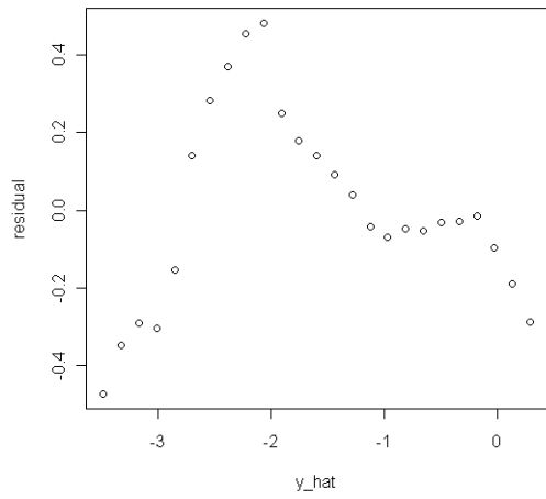
cglm_p(男_世代) : 配適値 vs 殘差
