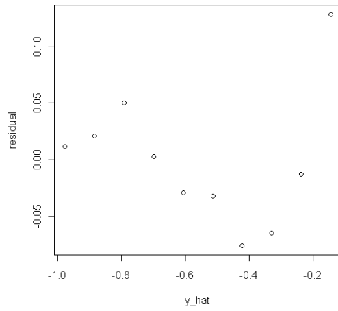
APC(男_年代) : 配適値 vs 殘差
