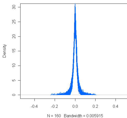
男性cglim_a-100次模擬的殘差機率密度函數
