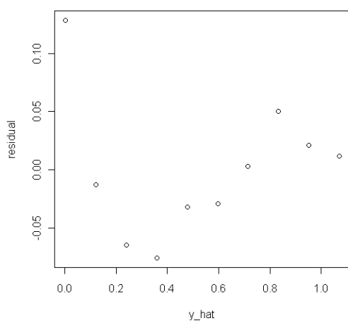
cglim_c(年代) : 配適値 vs 殘差
