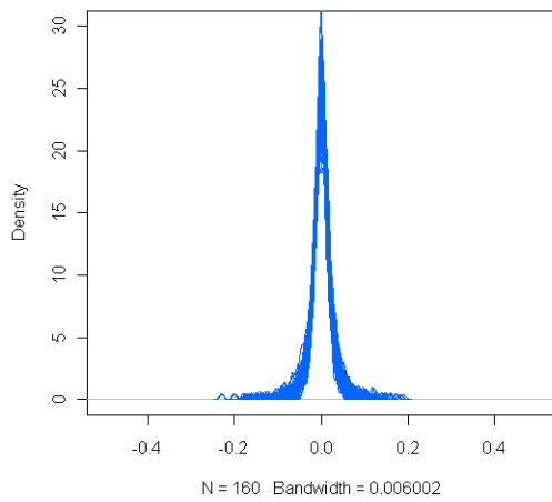
男性ar-100次模擬的殘差機率密度函數
