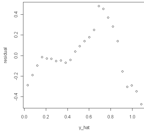
APC(世代) : 配適値 vs 殘差
