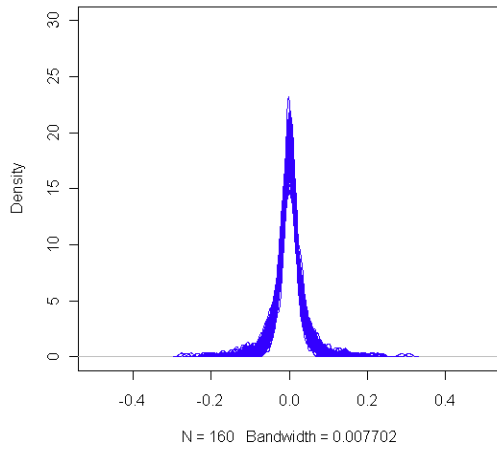
女性cglm_p-100次模擬的殘差機率密度函數
