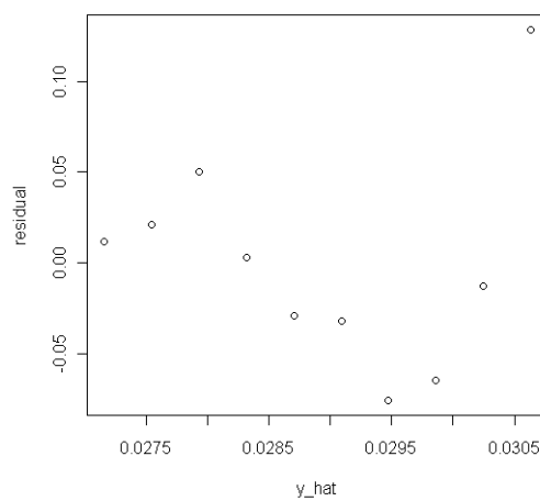
cglim_a(女_年代) : 配適値 vs 殘差
