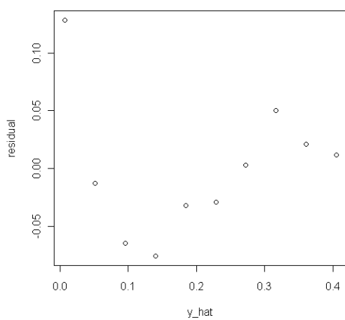
APC(年代) : 配適値 vs 殘差
