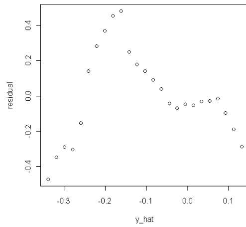
APC(男_世代) : 配適値 vs 殘差
