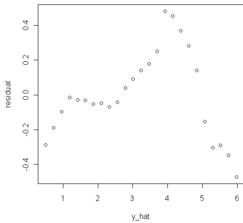
cglm_p(女_世代) : 配適値 vs 殘差
