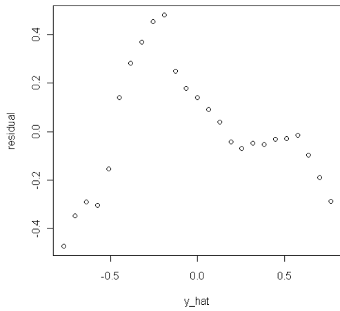
IE(女_世代) : 配適値 vs 殘差
