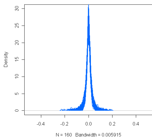
男性cglim_p-100次模擬的殘差機率密度函數
