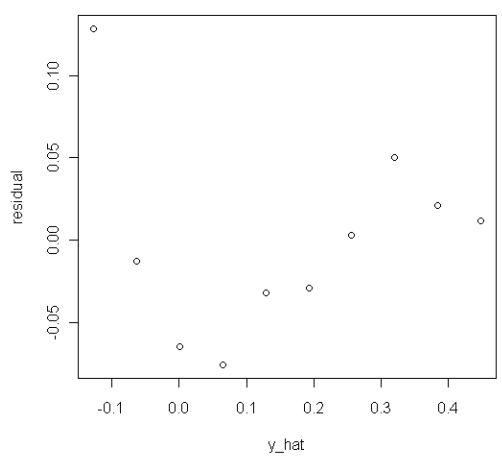
ACP(年代) : 配適値 vs 殘差
