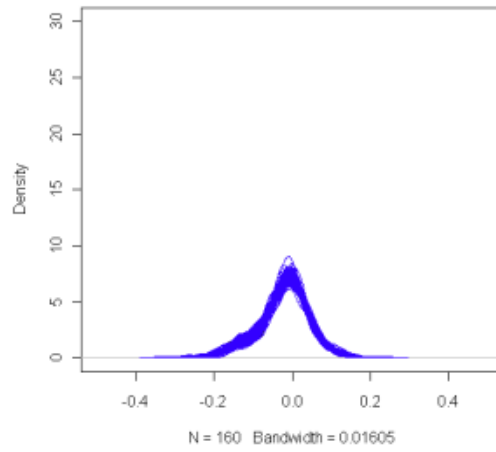
女性apc-100次模擬的殘差機率密度函數
