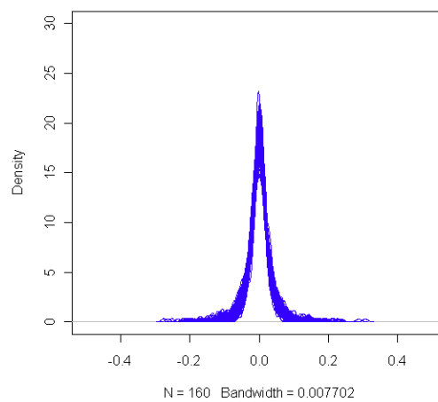
女性cglim_a-100次模擬的殘差機率密度函數
