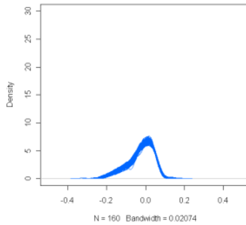
男性apc-100次模擬的殘差機率密度函數
