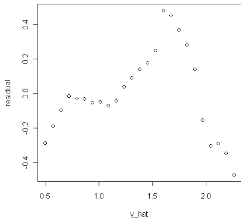
AR(世代) : 配適値 vs 殘差
