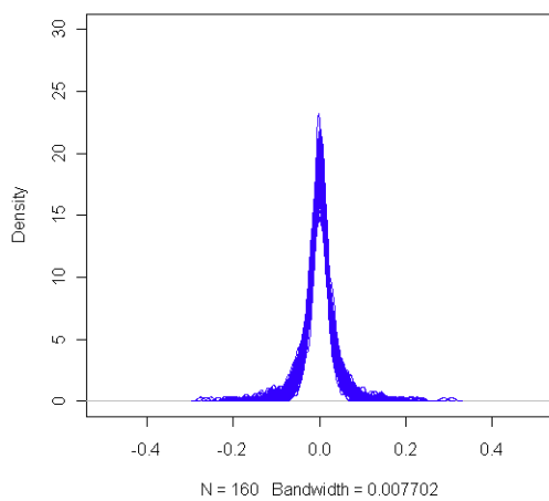
女性ie-100次模擬的殘差機率密度函數
