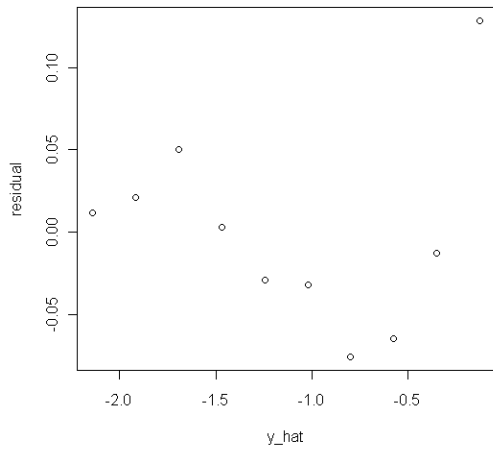
AR(年代) : 配適値 vs 殘差
