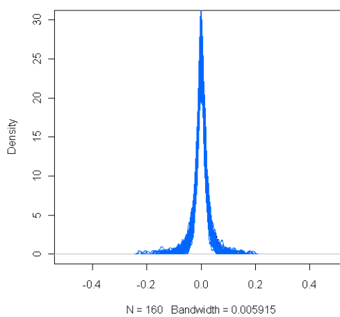
男性cglim_c-100次模擬的殘差機率密度函數
