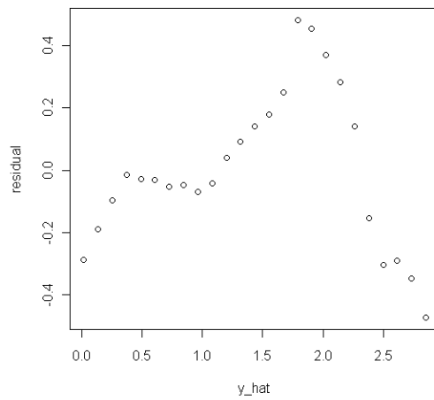
cglm_c(世代) : 配適値 vs 殘差
