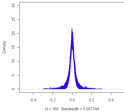
女性ar-100次模擬的殘差機率密度函數
