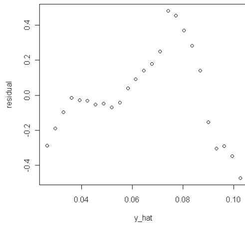
cglm_a(女_世代) : 配適値 vs 殘差
