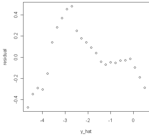
ACP(世代) : 配適値 vs 殘差
