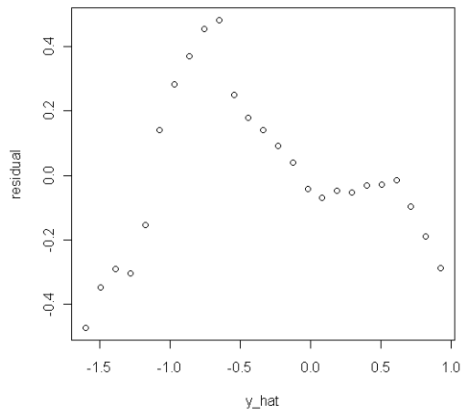
ACP(男_世代) : 配適値 vs 殘差
