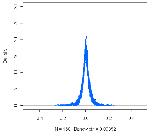
男性acp-100次模擬的殘差機率密度函數
