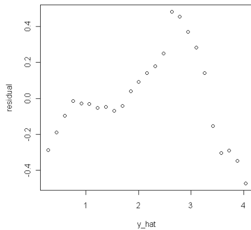
cglim_a(男_世代) : 配適値 vs 殘差
