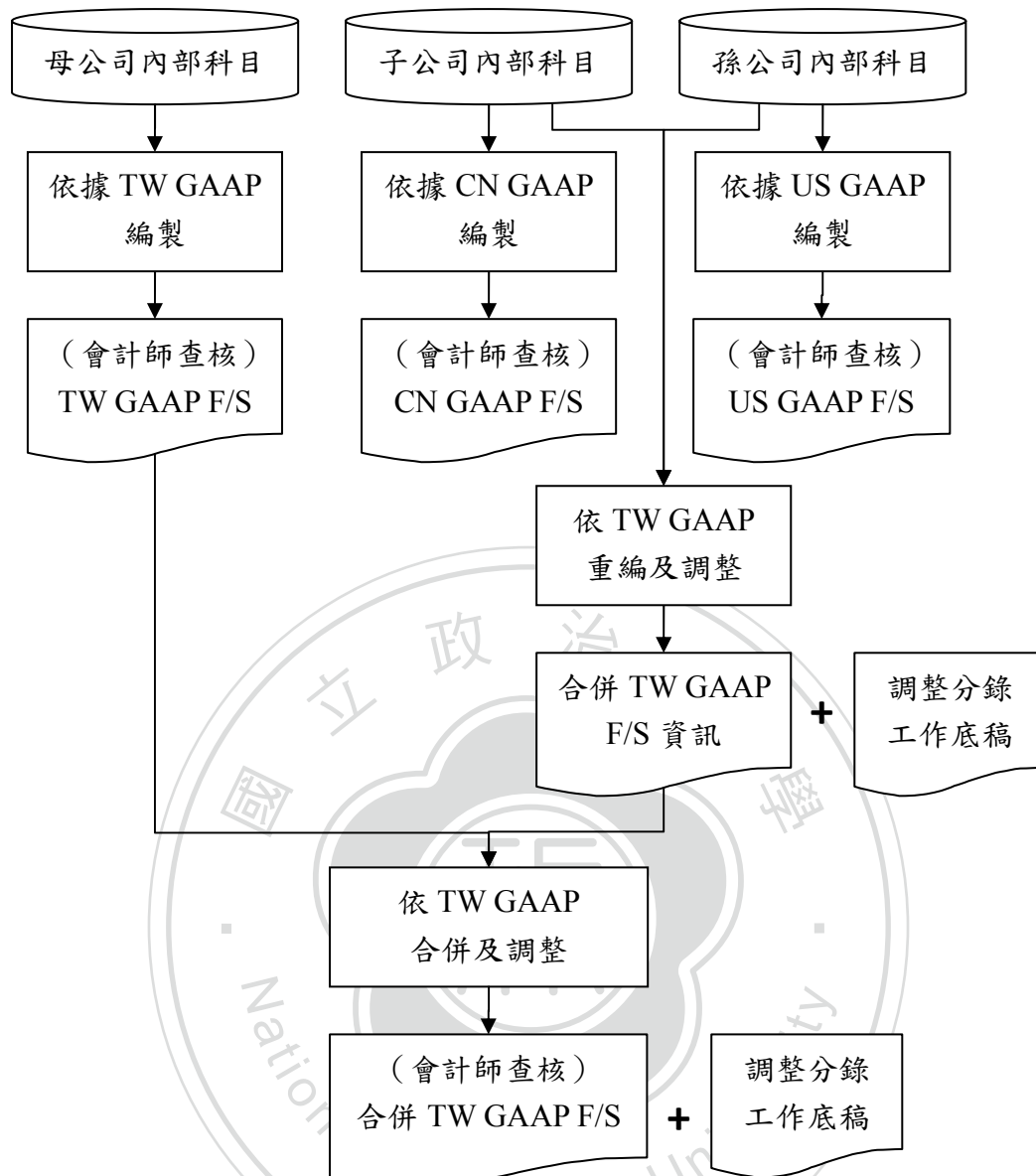
圖六 傳統企業財務報表資訊編製之流程圖
