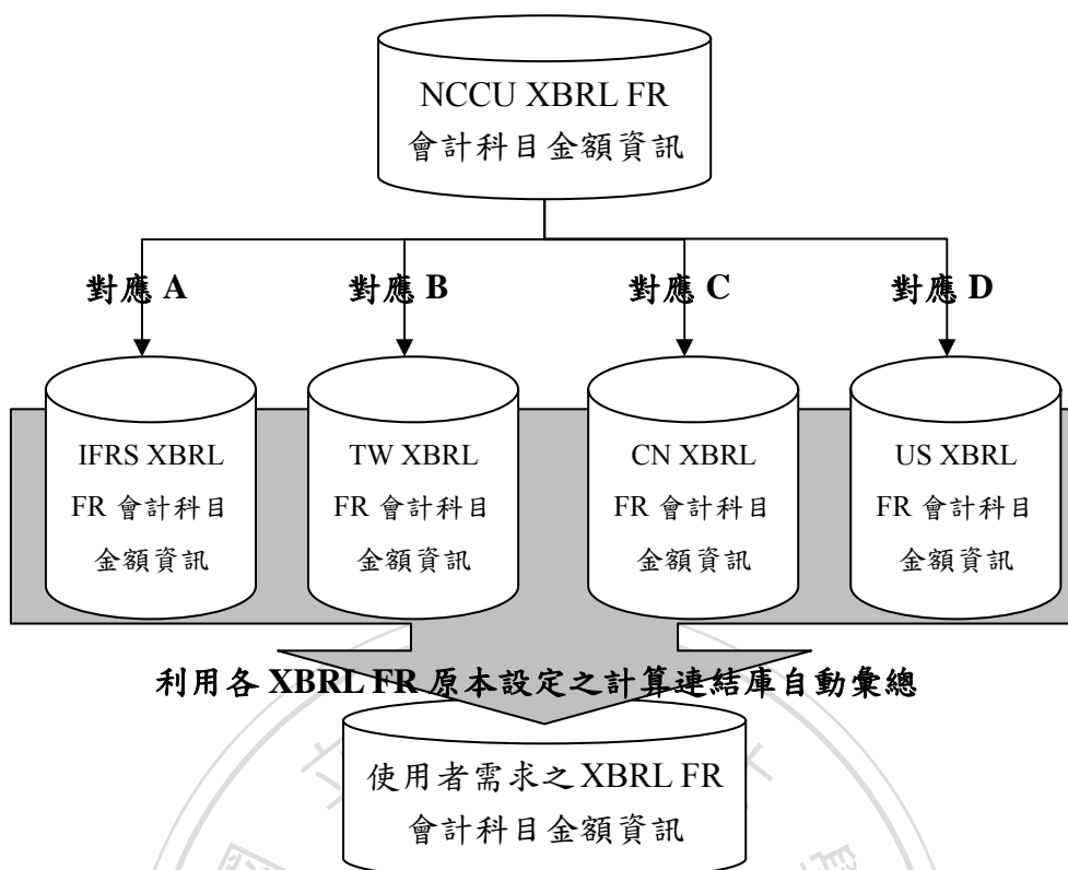
圖八 NCCU XBRL FR 協助企業財務資訊編製之架構
