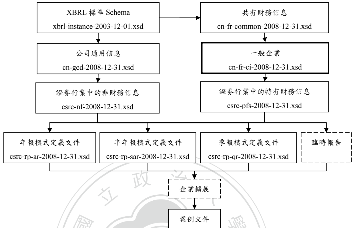
圖十二 中國大陸開放式企業報告分類標準套件結構（一般行業） 15
