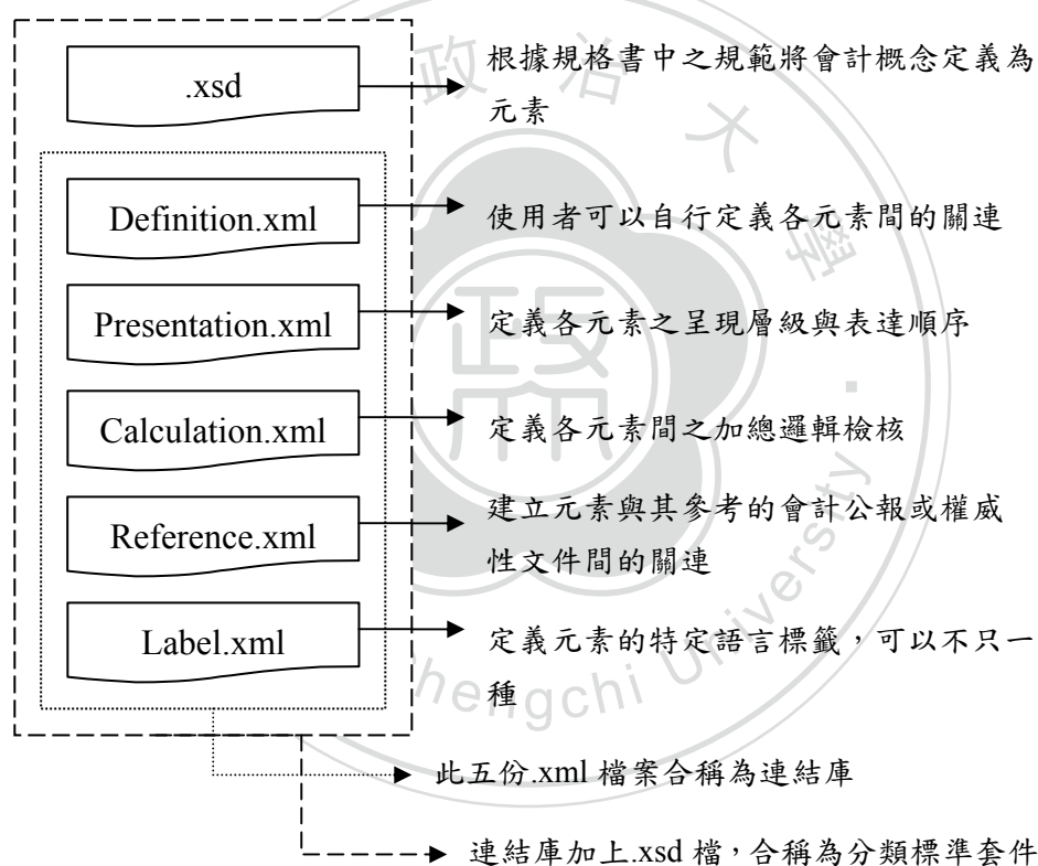
圖四 XBRL FR 分類標準套件之架構圖
