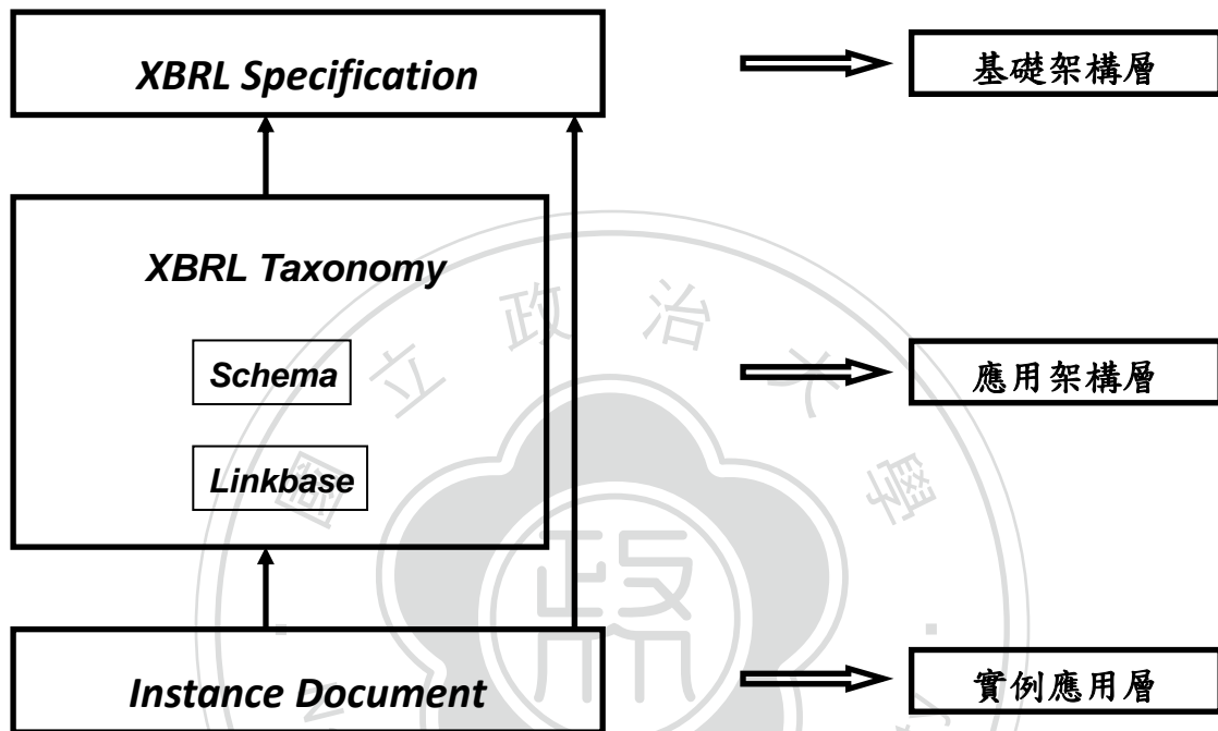
圖三 XBRL 技術架構圖
